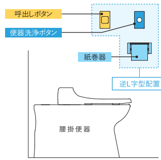
JIS規格になった操作系設備の配置ルール
