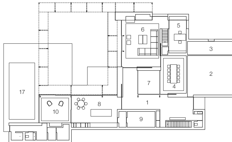
1階平面
