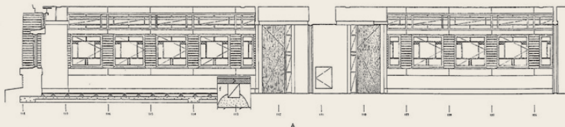
南側展開図
