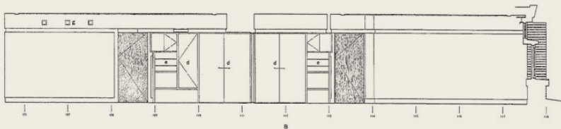
北側展開図
