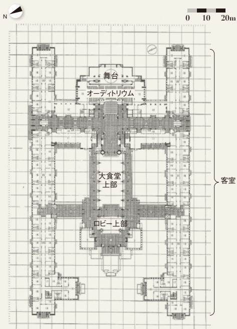
主階平面図
