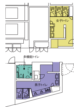
〔トイレ平面図〕
