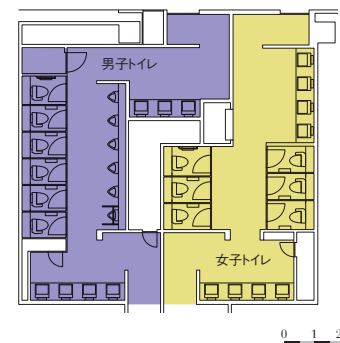
〔トイレ平面図〕
