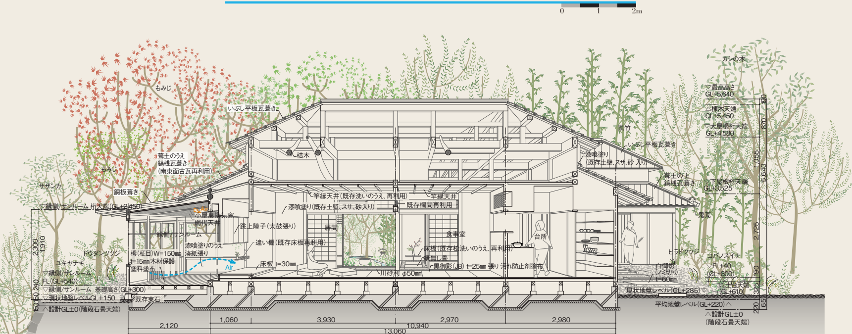
桁行断面図
