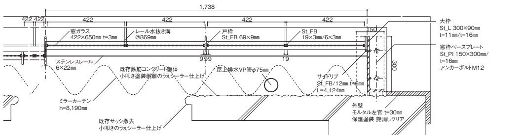
スチールサッシまわり平面詳細図
