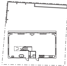
スチールサッシまわり平面詳細図
