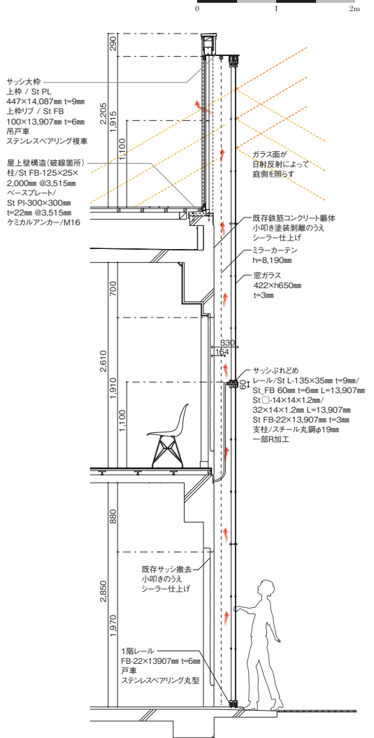
スチールサッシまわり断面詳細図
