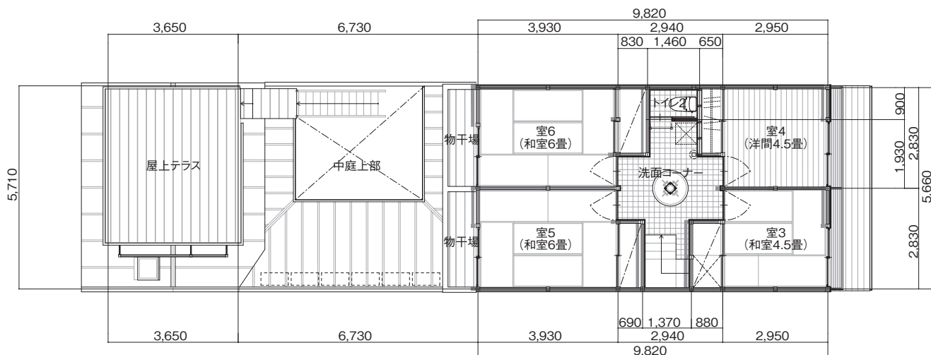
2階
