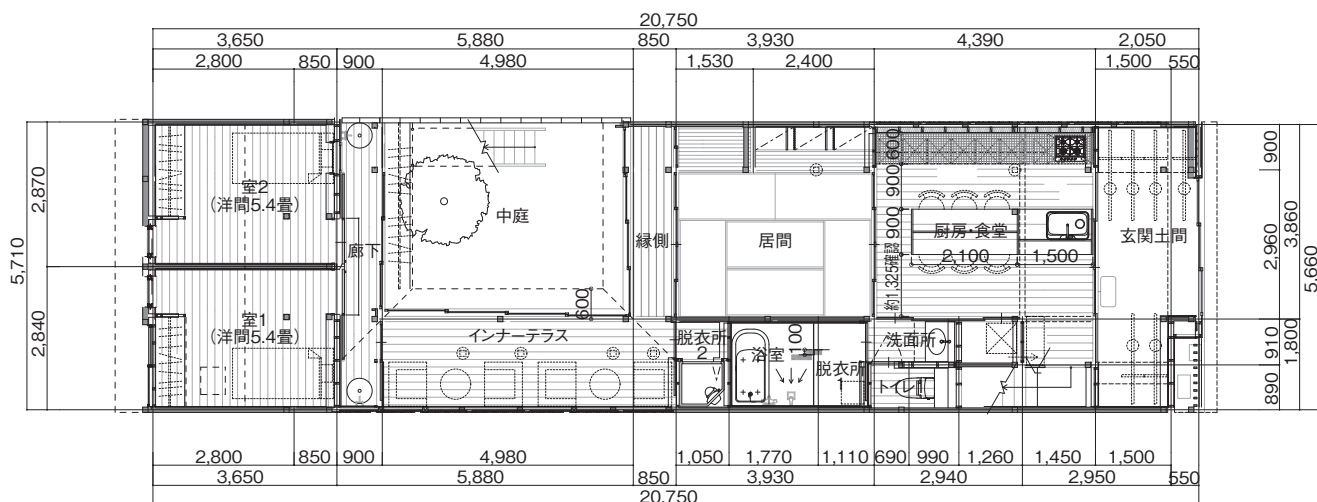
1階
