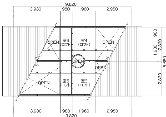
屋根階
