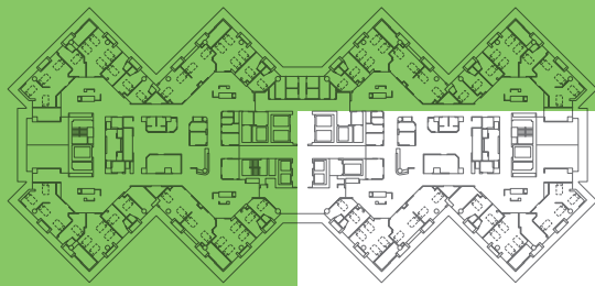
12F全体図
