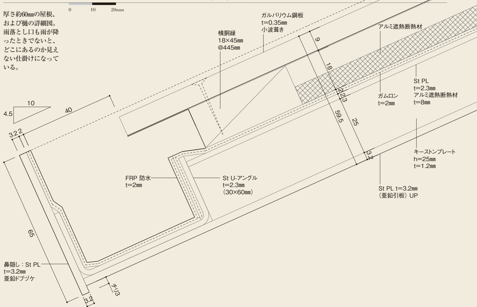
屋根詳細図
