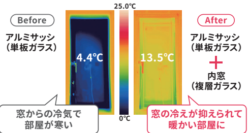
[サーモグラフィ撮影条件] 室内温度20.0°C / 室外温度-10.0°C YKK AP価値検証センター
