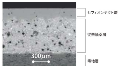
セフィオンテクト(新品) ※新品のセフィオンテクト便器の顕微鏡写真。 ※1µm=0.001mm
