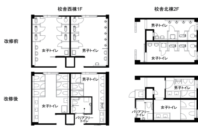
校舎棟トイレ図面
