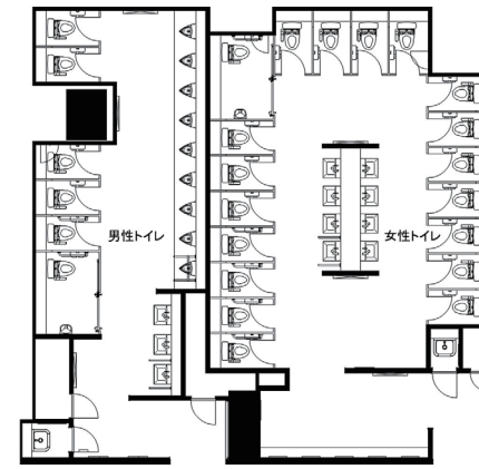
一般トイレ図面
