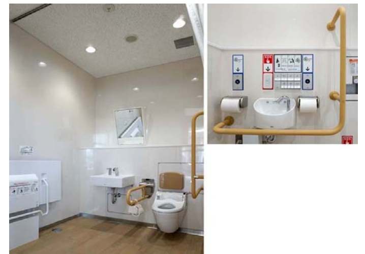
おむつ交換や衣服着脱のための収納式多目的シートを設置。大便器横には、座ったまま手指を洗うことができる壁掛手洗器を設置している。
