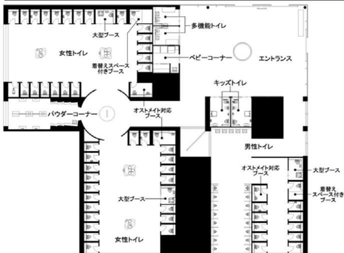
エントランスには、多機能トイレ、キッズトイレ、ベビーコーナーを配置。さらに、男女トイレ内にはオストメイト対応ブースなどの個別機能を備えたブースを設けることにより、トイレ全体の機能分散を図っている。
