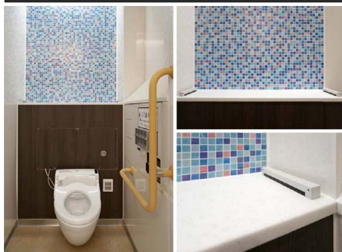
男性トイレの大便器ライニング上に、忘れ物を感知するセンサーを設置。荷物を置いた状態でブース扉を開けて出ようとする時、荷物確認のアナウンスが流れる仕組みになっている。
