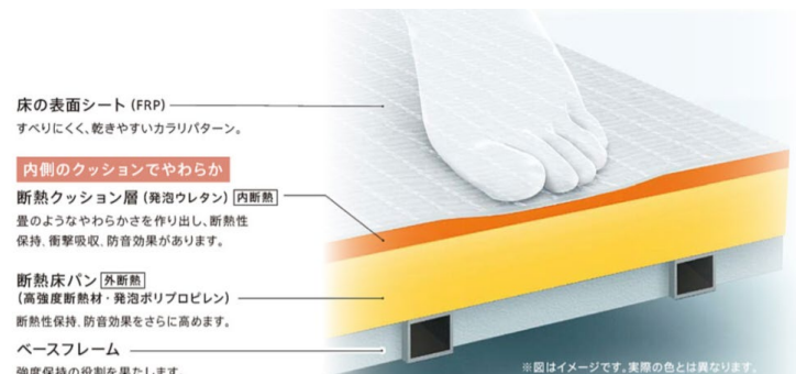
お掃除ラクラクほっカリ床の構造
